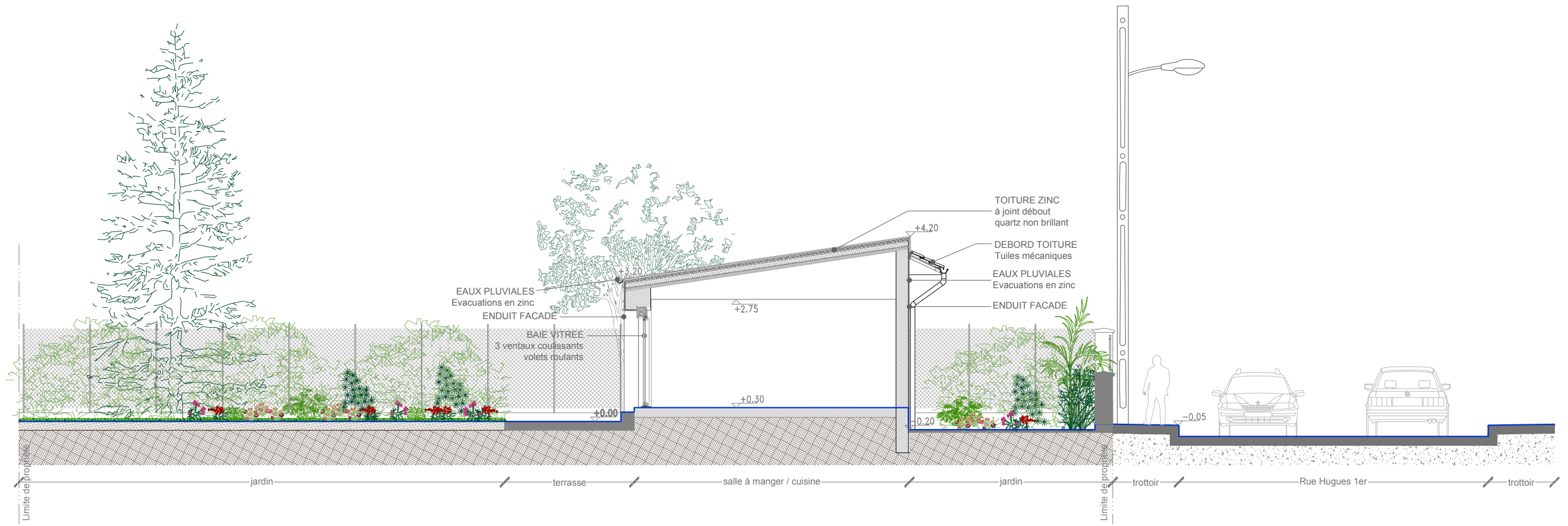
ETAT EXISTANT - Coupe de Terrain TT
