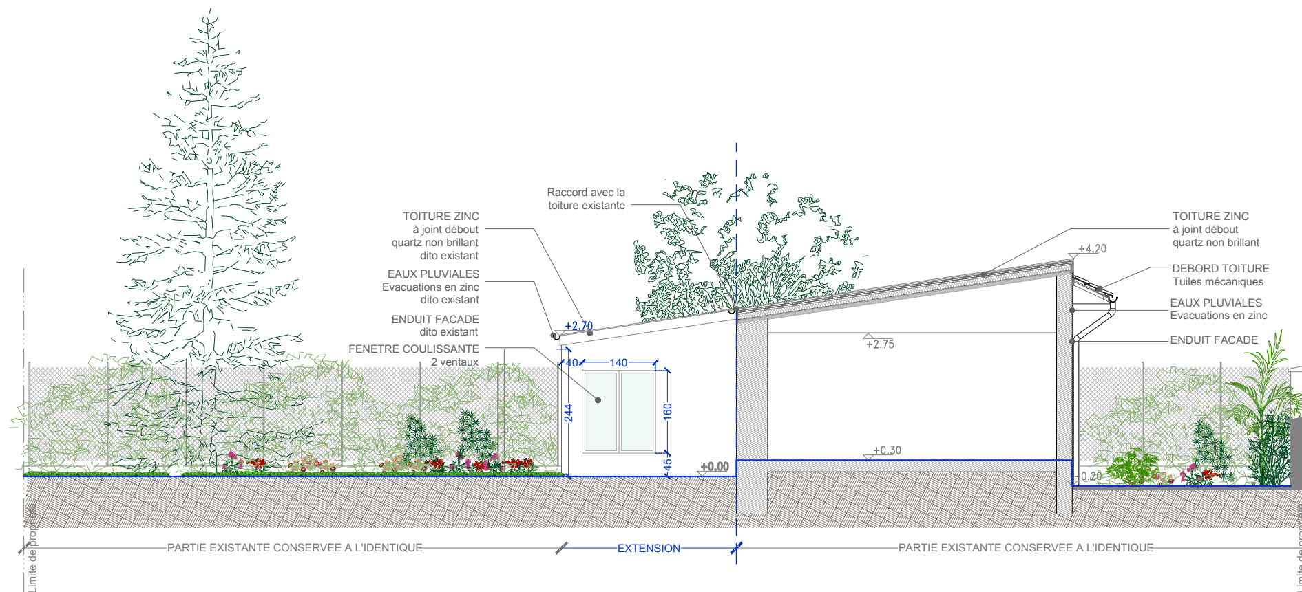
ETAT PROJETE - Façade Nord-Ouest - Coupe AA
