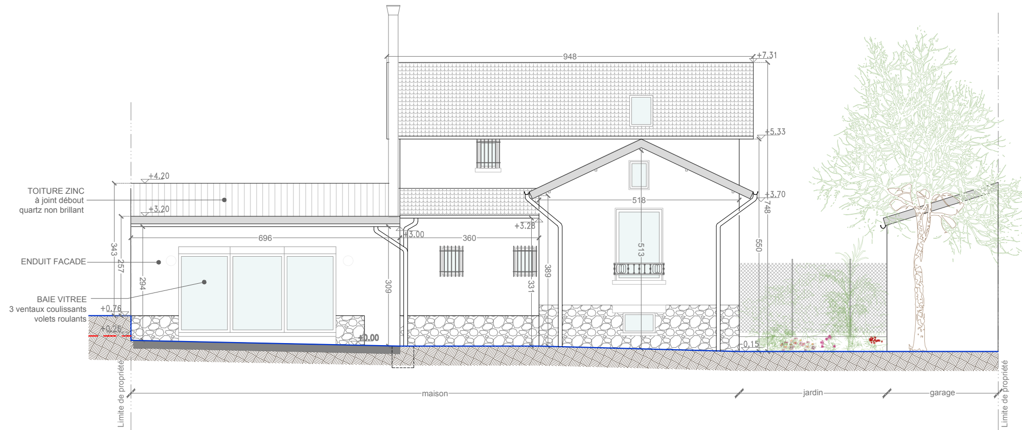
ETAT EXISTANT - Façade Nord-Est
