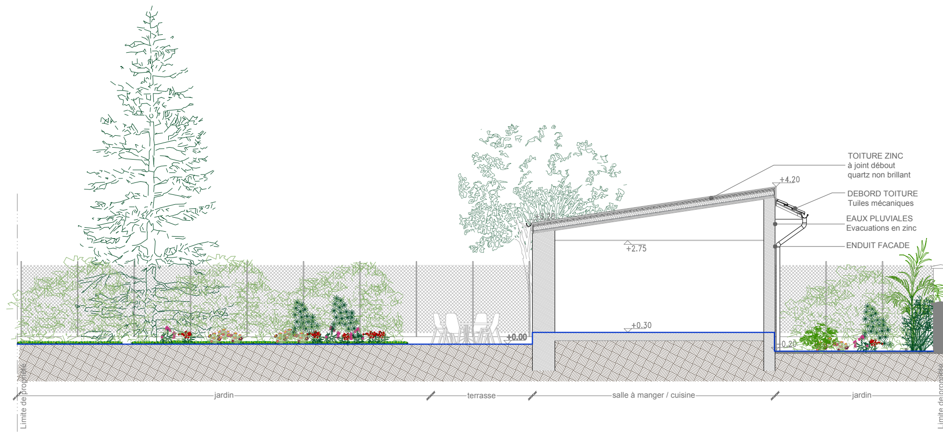
ETAT EXISTANT - Façade Nord-Ouest - Coupe AA
