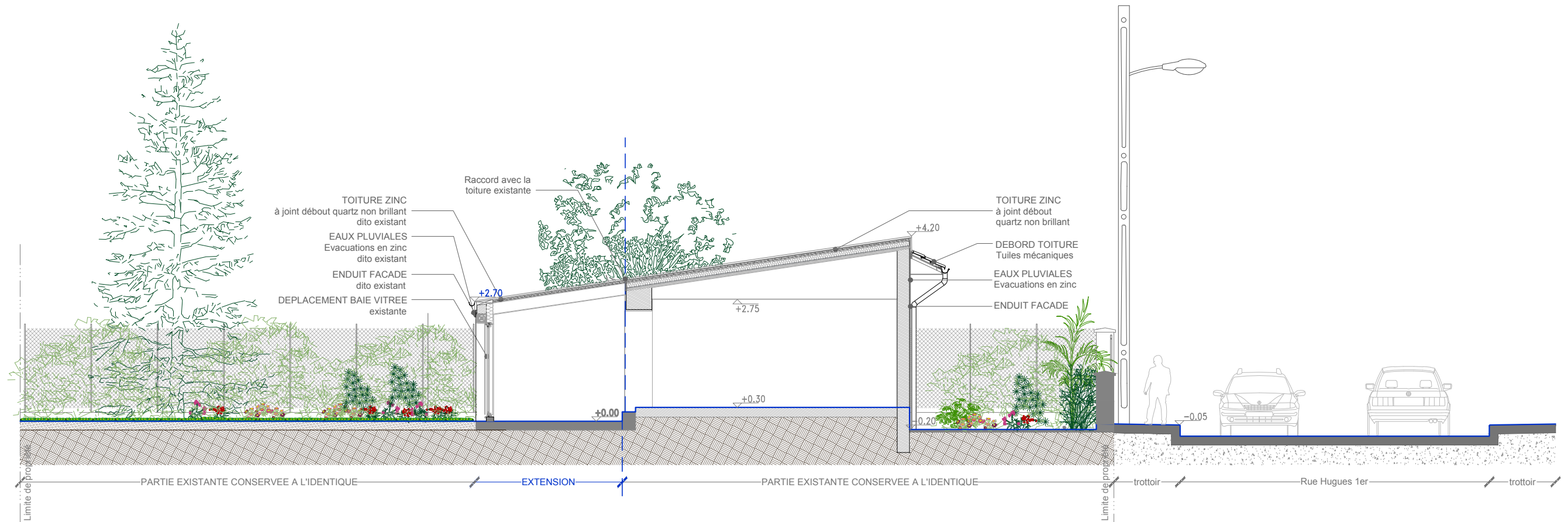
ETAT PROJETE - Coupe de Terrain TT
