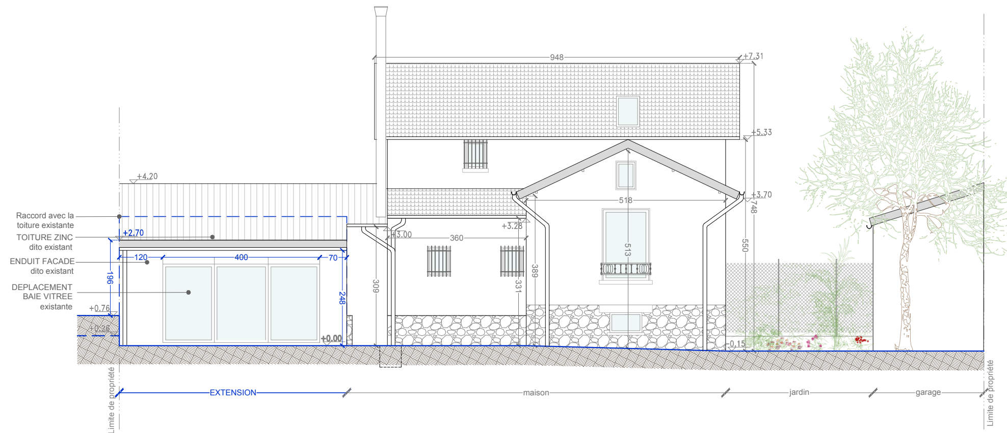
ETAT PROJETE - Façade Nord-Est
