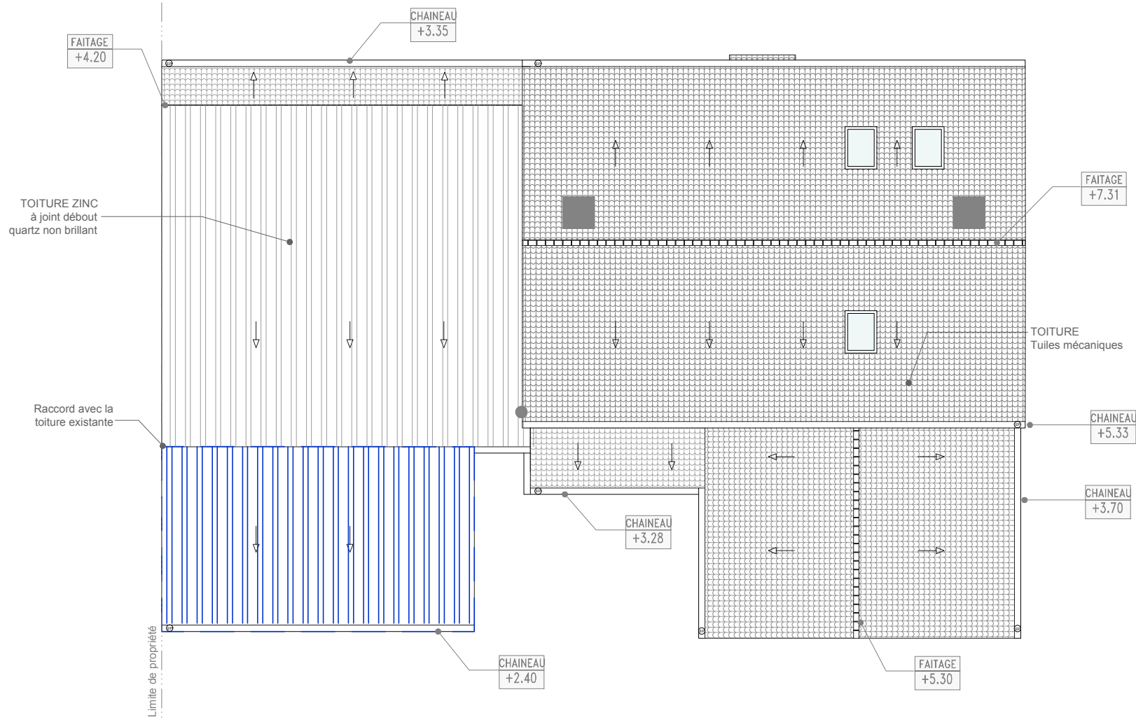
ETAT PROJETE - Toiture
